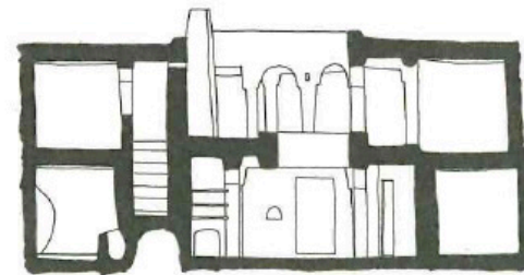
coupe B
