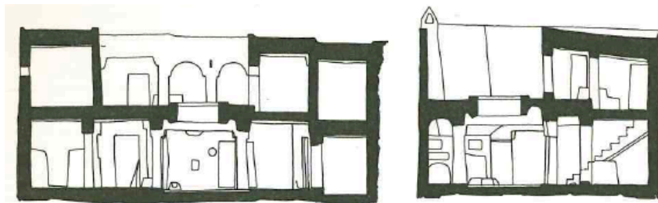
coupe A
